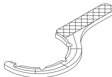
排水金具締付け工具
